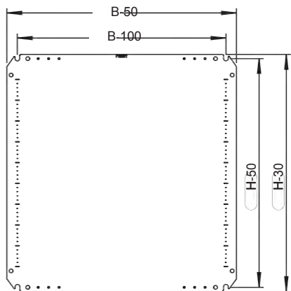
Összeszerelési nézet
