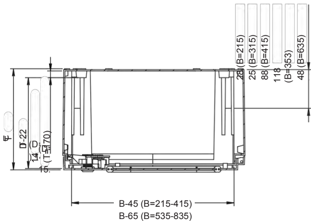
KITERJEDÉS A-A
