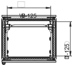
Felülnézeti metszet
