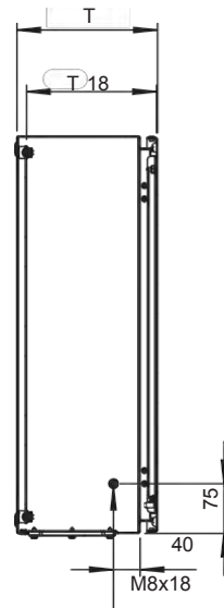
Oldalnézet
