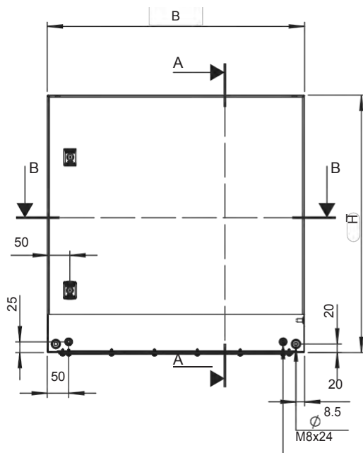
Felülnézeti metszet
