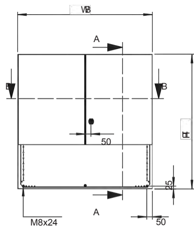
Előlnézet
