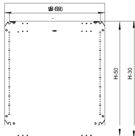
Összeszerelési nézet
