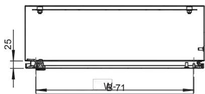
KITERJEDÉS B-B
