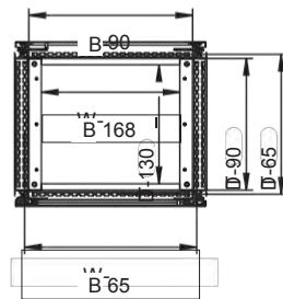
Felülnézeti metszet (alaplemez nélkül)
