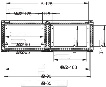
KITERJEDÉS B-B
