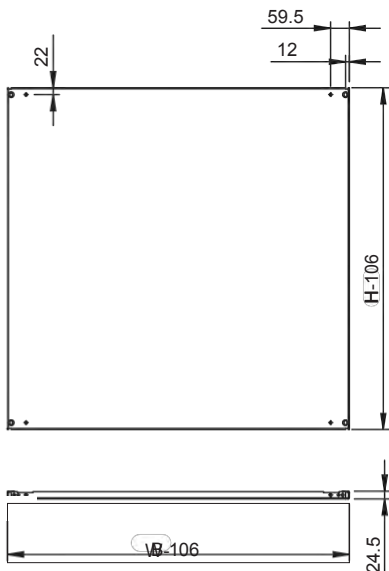
KITERJEDÉS A-A
