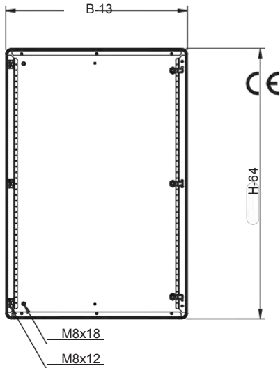
Ajtó belső metszet
