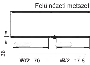
KITERJEDÉS B-B
