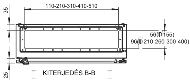
Felülnézeti metszet
