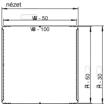
Összeszerelési nézet
