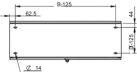
Felülnézeti metszet (alaplemez nélkül)
