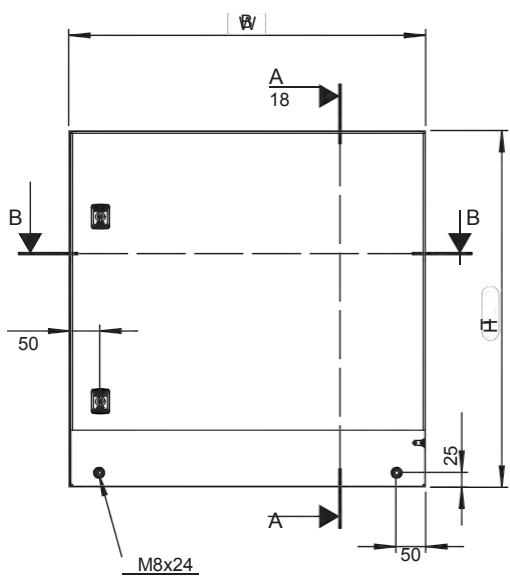
Előlnézet
