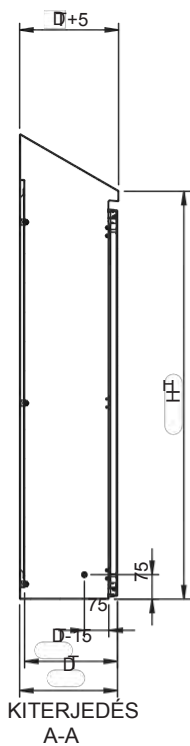
Oldalnézet
