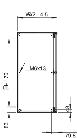
Összeszerelési nézet
