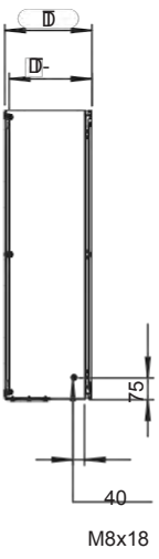
Oldalnézeti metszet
