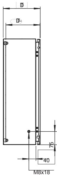
KITERJEDÉS A-A
