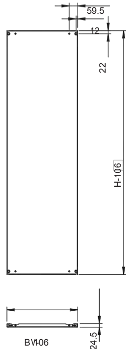
Összeszerelési nézet
