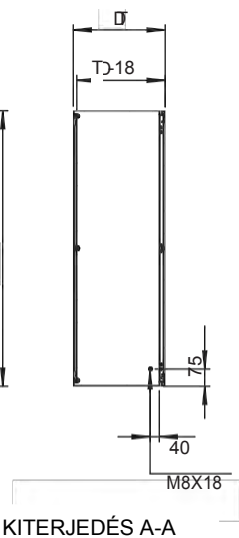
Oldalnézeti metszet
